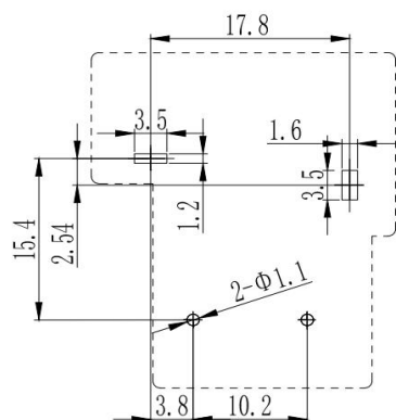
安装尺寸图
