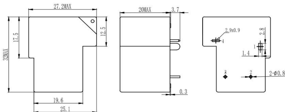
外形图
